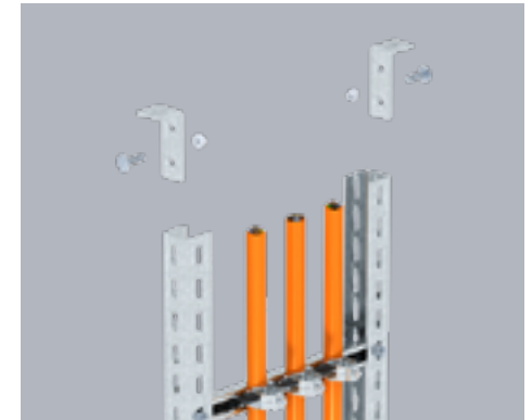
Deckenbefestigung mit Montagewinkeln Ceiling mounting with mounting brackets
