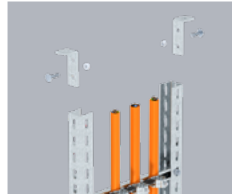
Deckenbefestigung mit Kopfplatten Ceiling mounting with head plates
