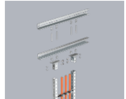
Direkte Montage der Steigeleiter Typ SLM50C40F ... an Massivwand Direct mounting of the vertical ladder type SLM50C40F ... on solid wall
