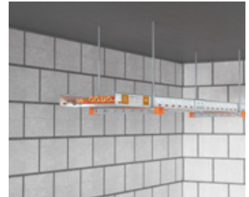
Deckenmontage mit Querprofil
