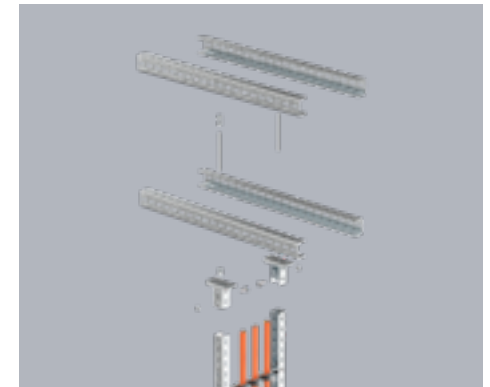
Deckenbefestigung mit Kopfplatten an rechtwinklig angeordneten U-Profilen Ceiling mounting with head plates on profiles arranged at right angle
